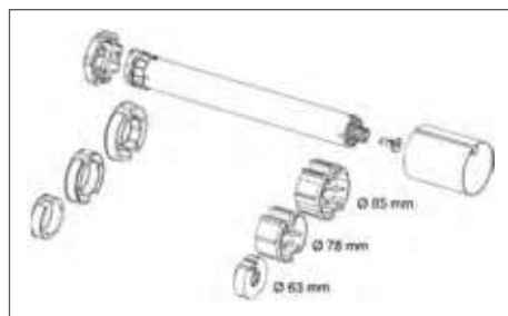
Afbeelding 1: Voorbeelden van verschillende asontrekken
