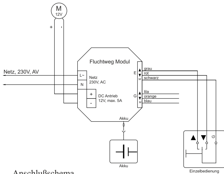
Anschlussschema
