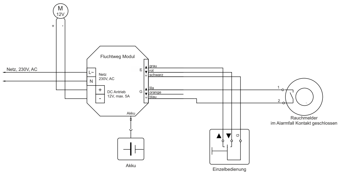
Anbindung an einen Rauchmelder
