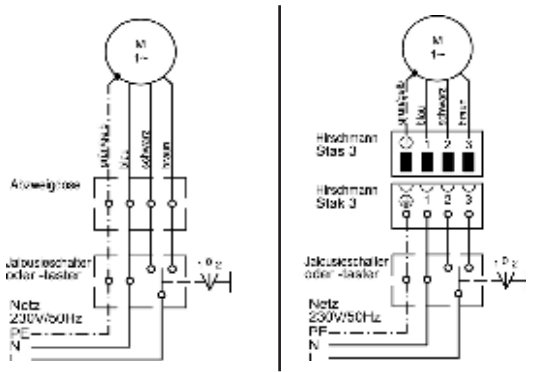
Fig. 4 Schaltbild VariEco S-K mit 230 V / 50 Hz
