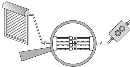
Fig. 5 Anschluss für Montagekabel
