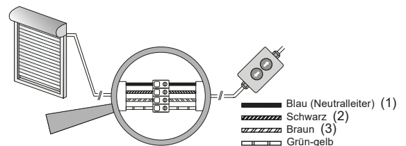
Fig. 6 Anschluss für Montagekabel
